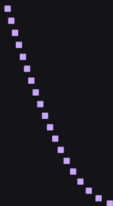
Verlet Rope
